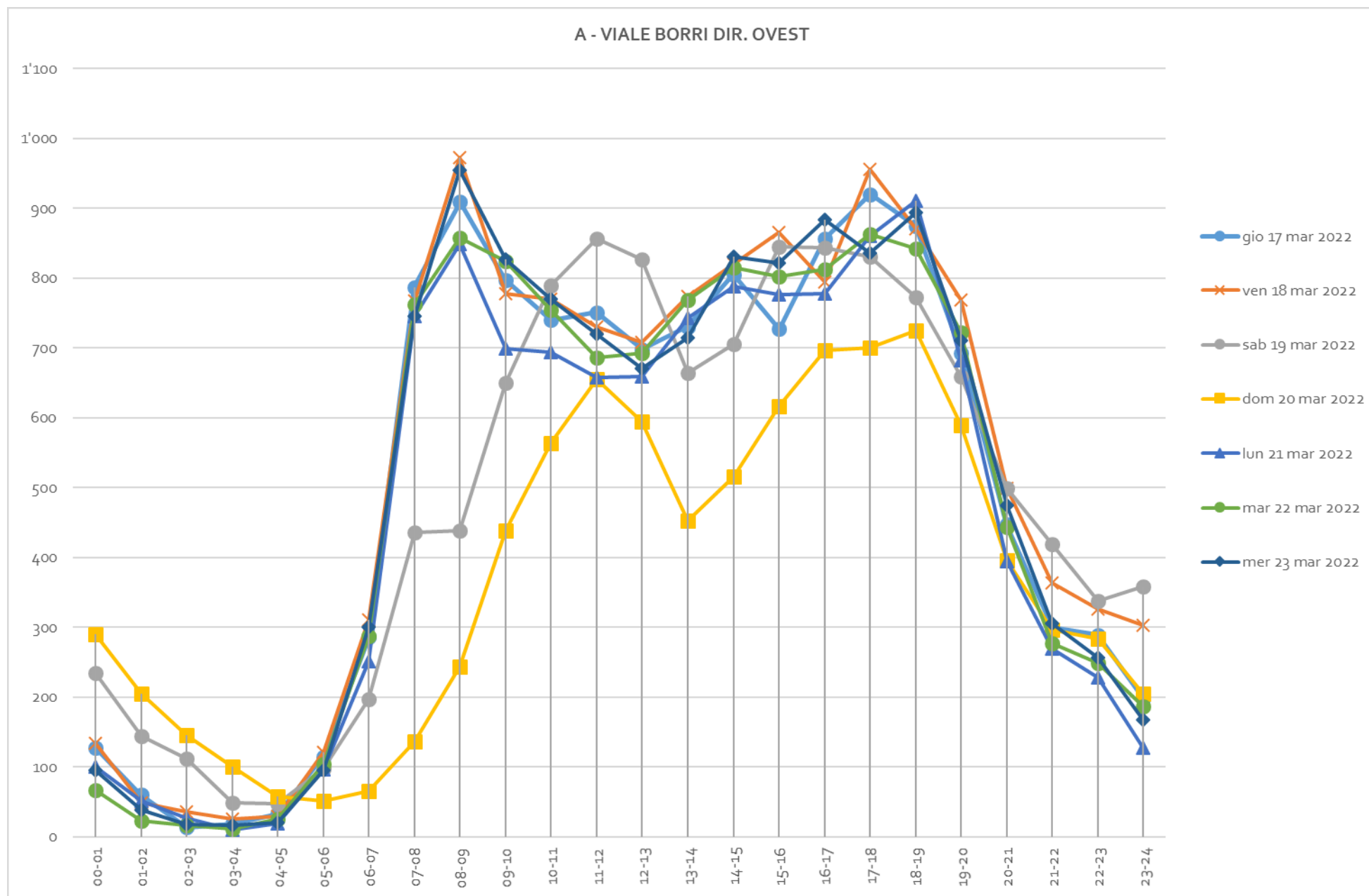
Grafico 2 – Sezione A – Flussi complessivi per fascia oraria e giorno della settimana – direzione ovest
