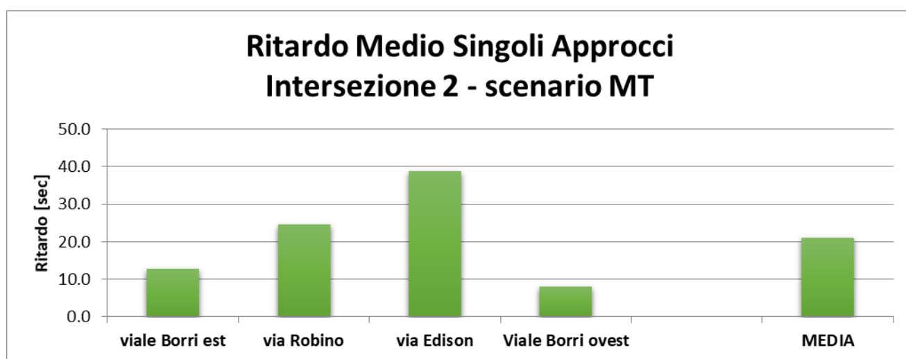
Grafico 015 – Scenario di intervento di MT – intersezione 2 – Perditempo medio complessivo
