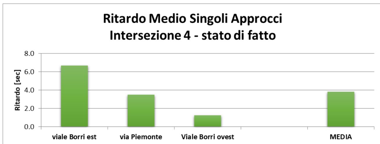
Grafico 025 – Scenario attuale – intersezione 4 – Perditempo medio complessivo
