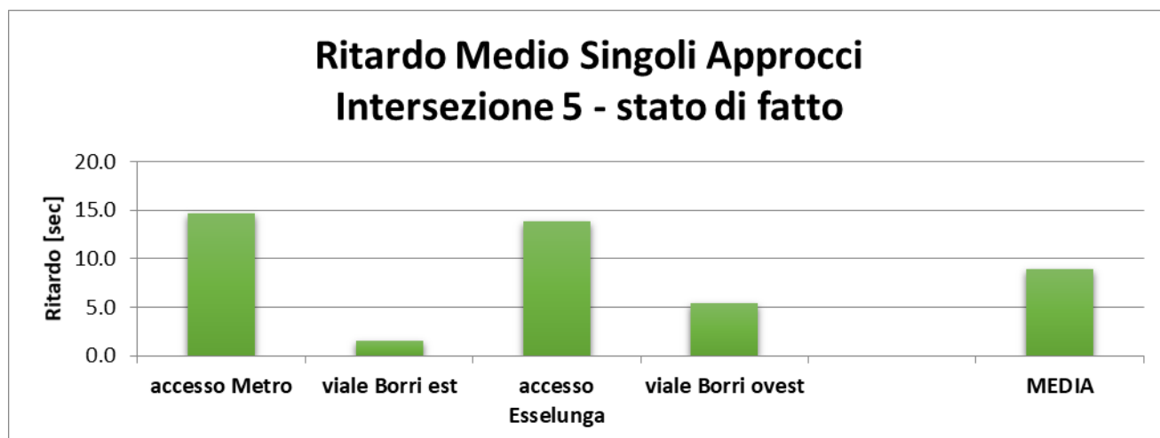
Grafico 031 – Scenario attuale – intersezione 5 – Perditempo medio complessivo
