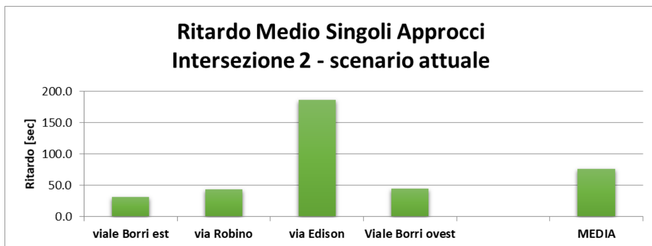
Grafico 13 – Scenario attuale – intersezione 2 – Perditempo medio complessivo
