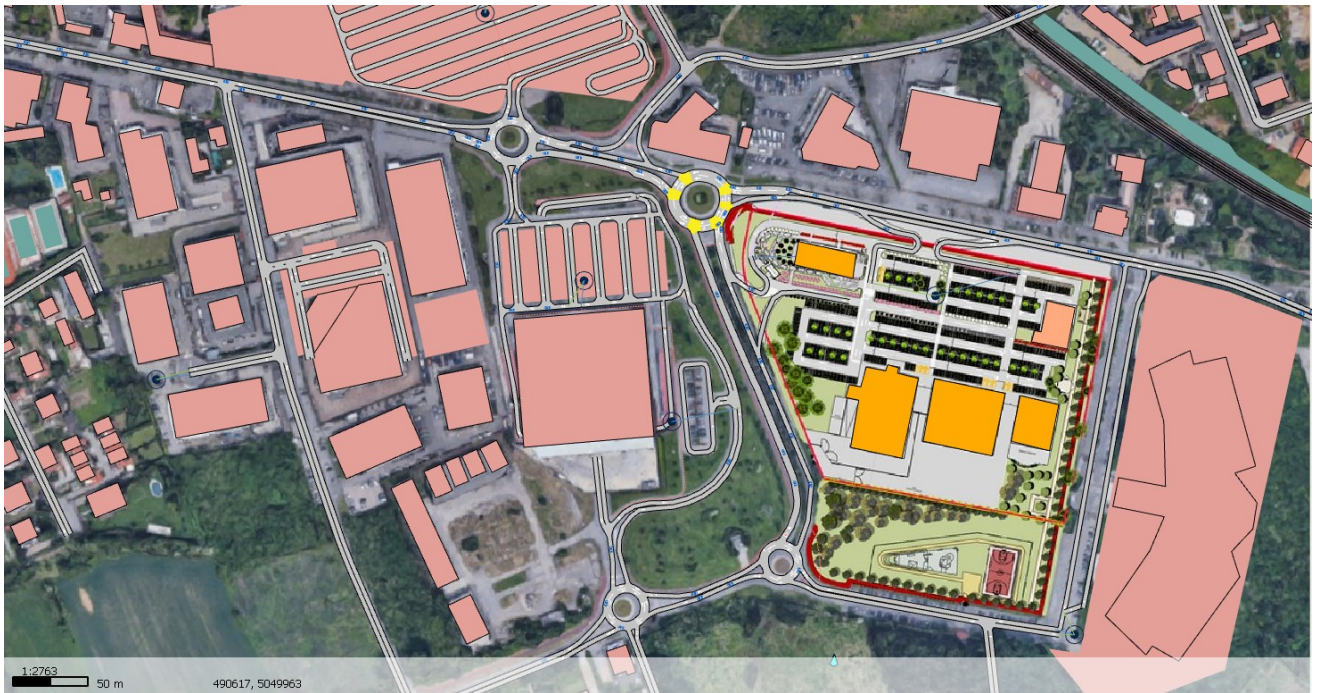
Figura 73 - Scenario di intervento MT – Istantanea dopo 40 minuti di simulazione
