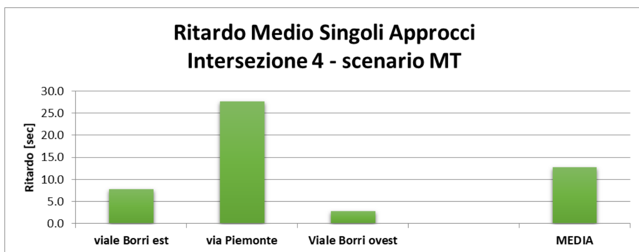
Grafico 027 – Scenario di intervento di MT – intersezione 4 – Perditempo medio complessivo
