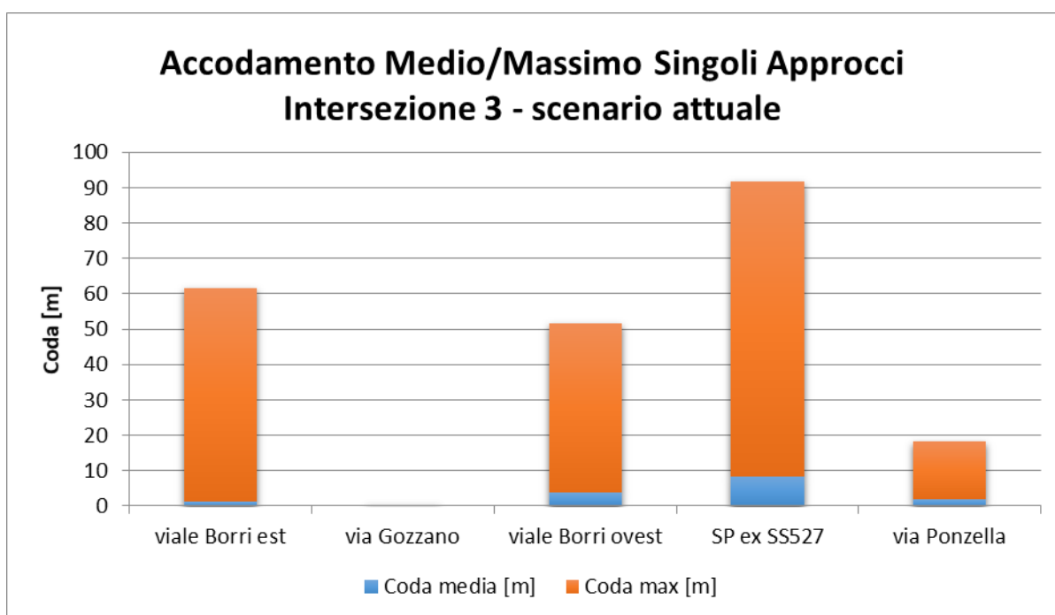
Grafico 022 – Scenario attuale – intersezione 3 – accodamento medio e massimo
