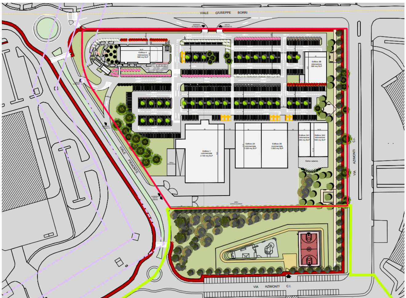
Figura 47 – Planimetria di progetto
