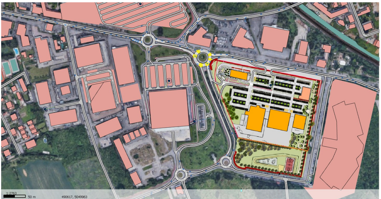
Figura 66 - Scenario di intervento MT – Istantanea dopo 5 minuti di simulazione
