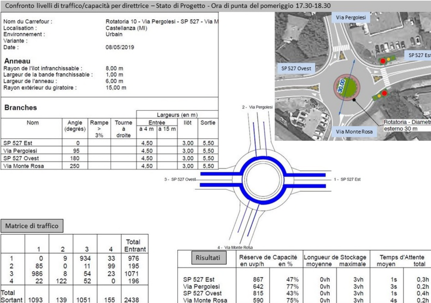
Figura 7.0.6 – Risultati dell'intersezione Via Pergolesi-Via Monte Rosa-Sp 527
