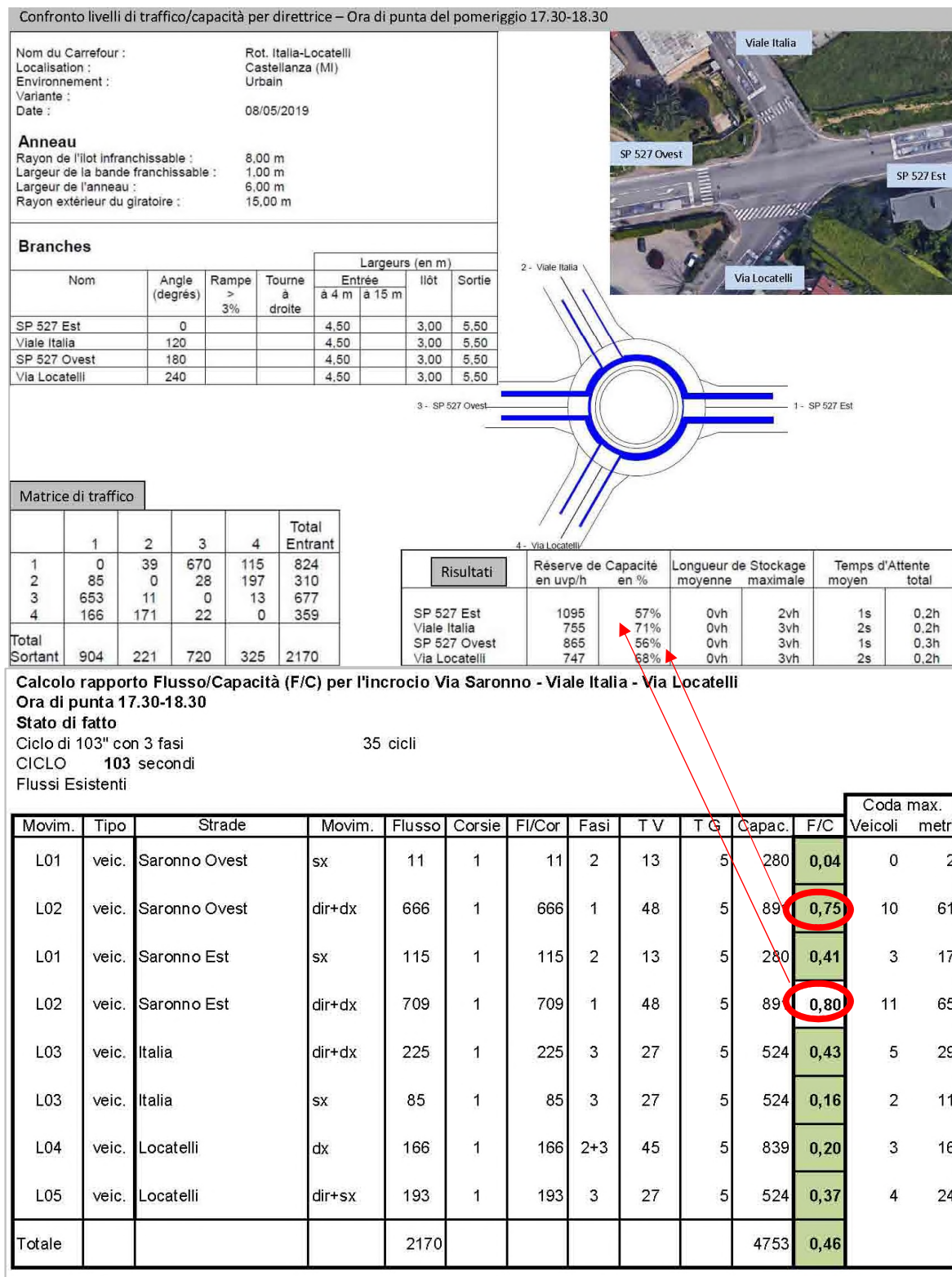
Figura 7.0.7b – Confronto della riserva di capacità tra un'intersezione semaforizzata e una rotonda Ora di punta del Pomeriggio
