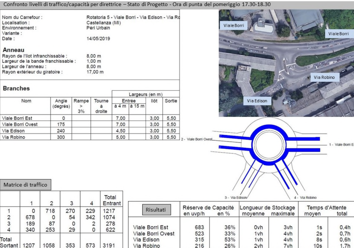
Figura 7.0.2 – Risultati dell'intersezione Viale Borri-Via Edison-Via Robino
