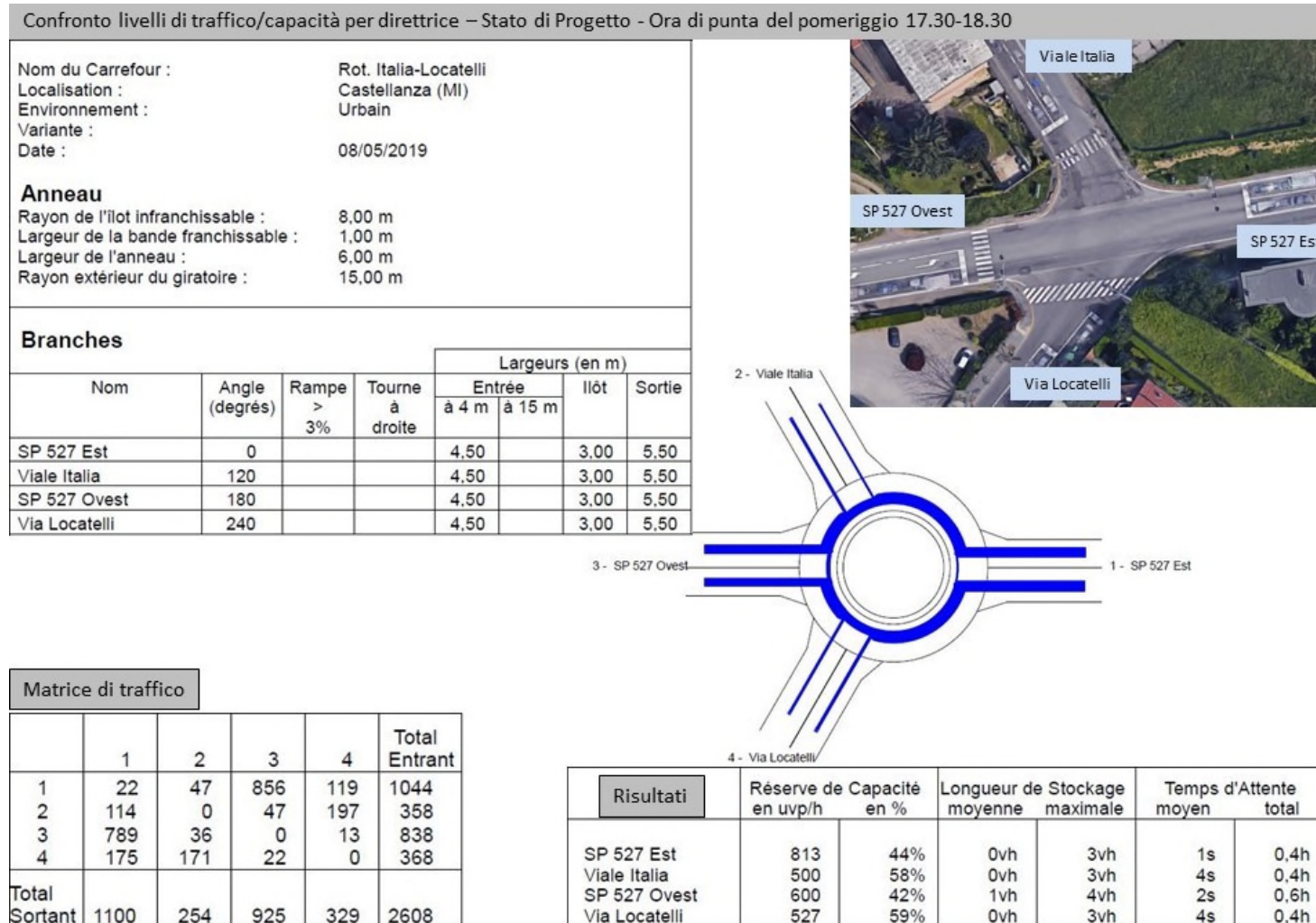
Figura 7.0.4 – Risultati dell'intersezione Via Locatelli-Viale Italia-sp 527
