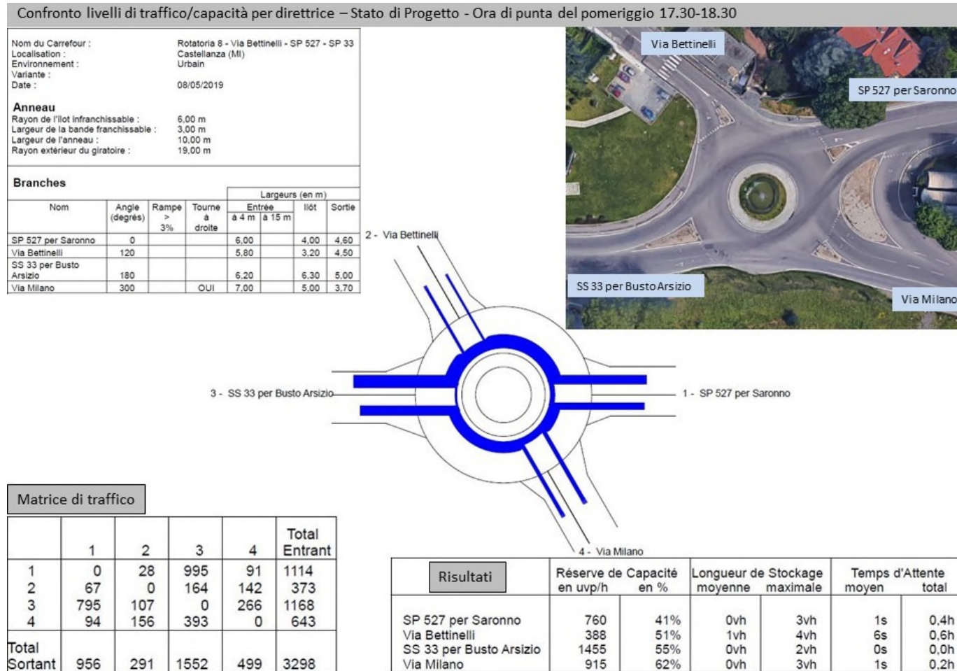
Figura 7.0.1 – Risultati dell'intersezione Via Bettinelli-Via Milano-SP 527
