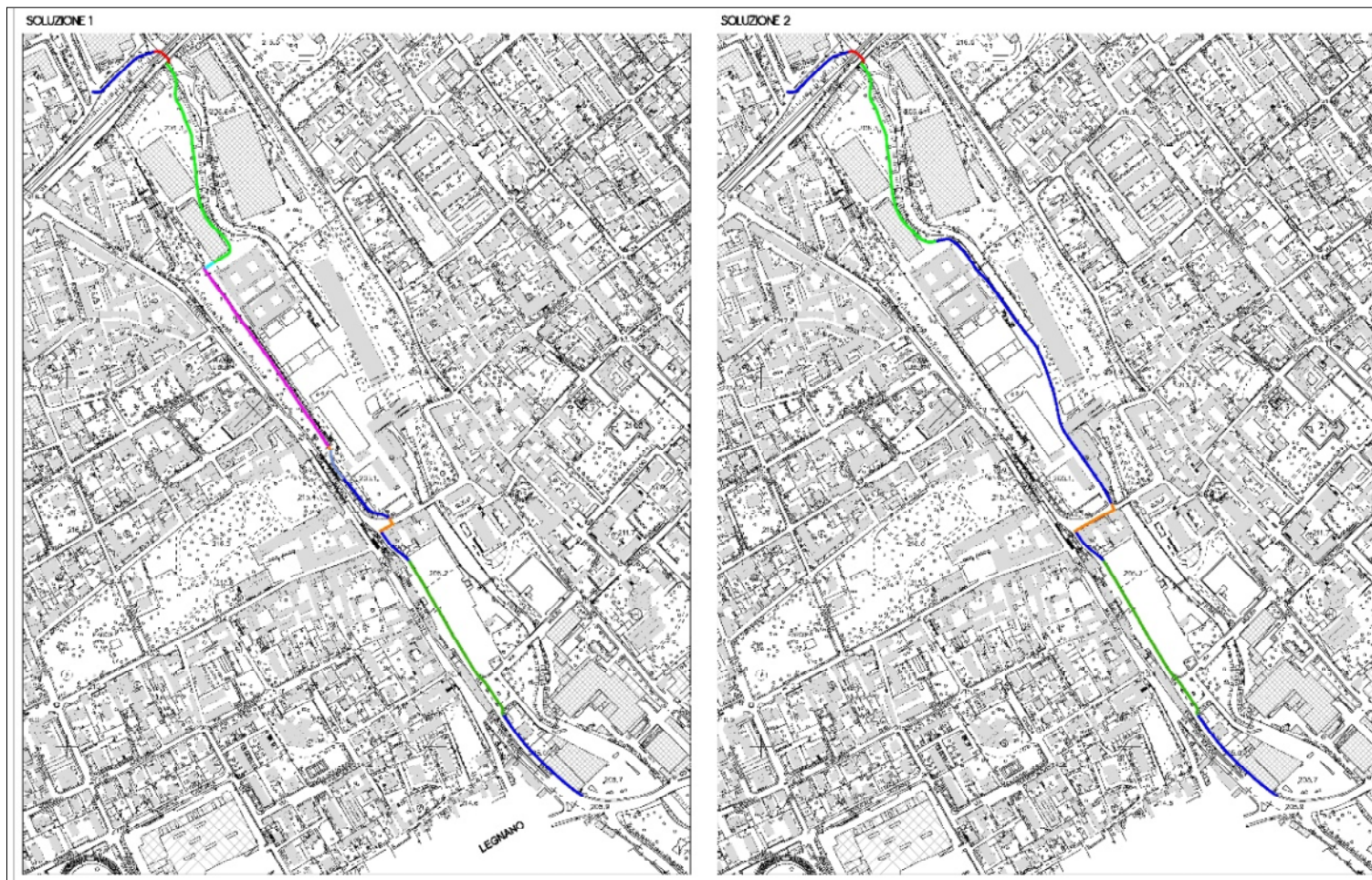
Figura 5.1.2 – Progetto per la realizzazione di una pista ciclabile nel territorio del Comune di Castellanza
