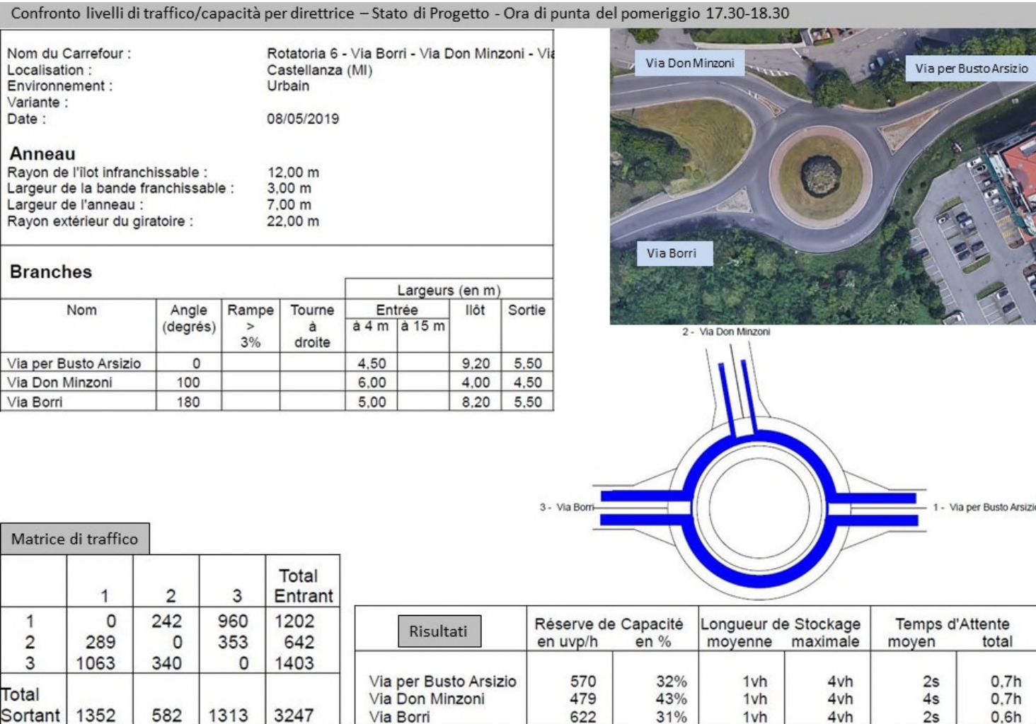
Figura 7.0.3 – Risultati dell'intersezione Via Don Minzoni-Via Borri-Via per BustoArsizio
