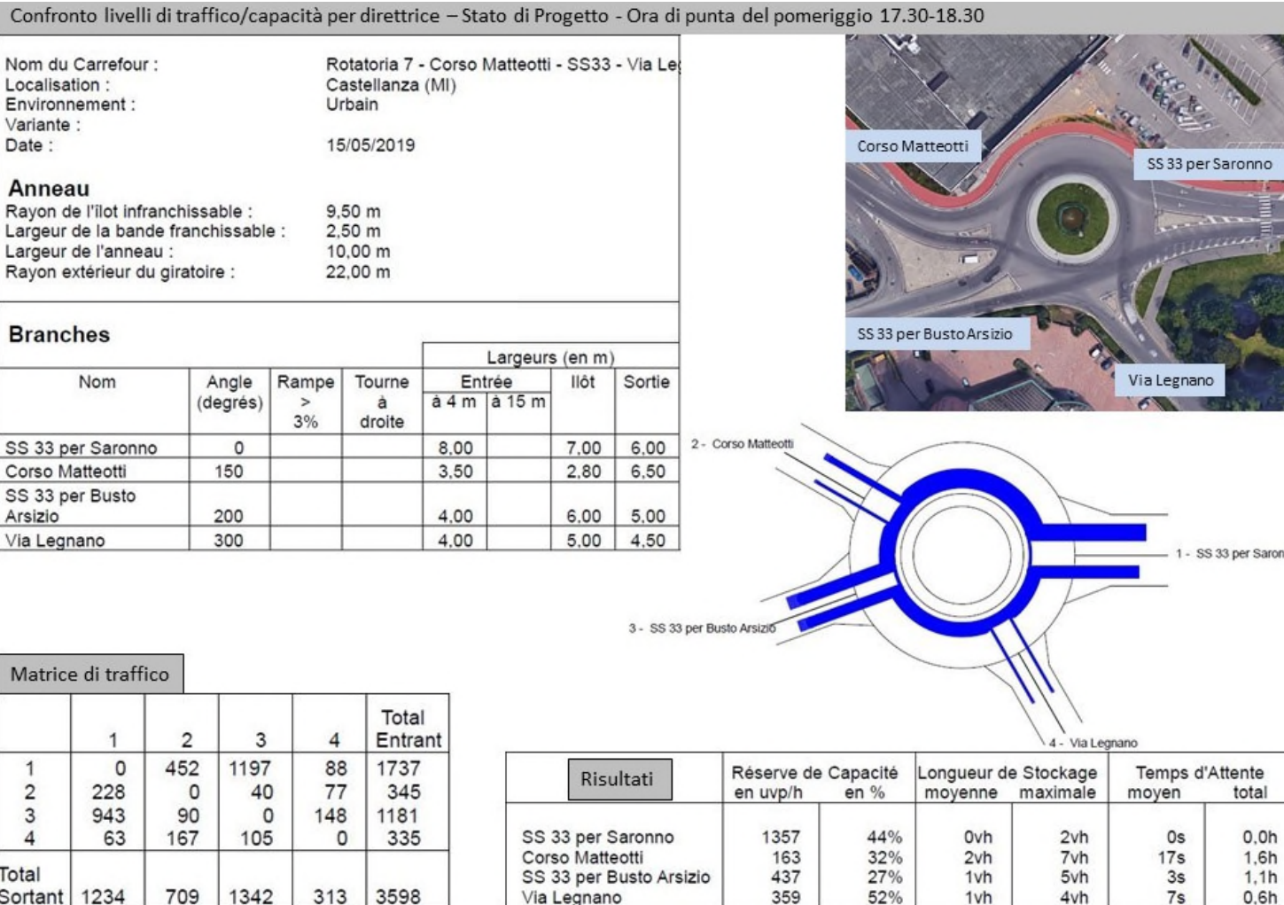
Figura 7.0.5 – Risultati dell'intersezione Corso Matteotti-Via Legnano-SS 33
