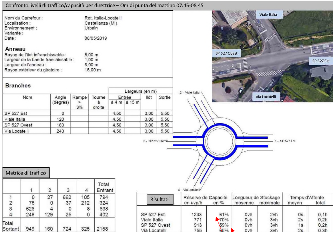
Figura 7.0.7a – Confronto della riserva di capacità tra un'intersezione semaforizzata e una rotonda Ora di punta del mattino
