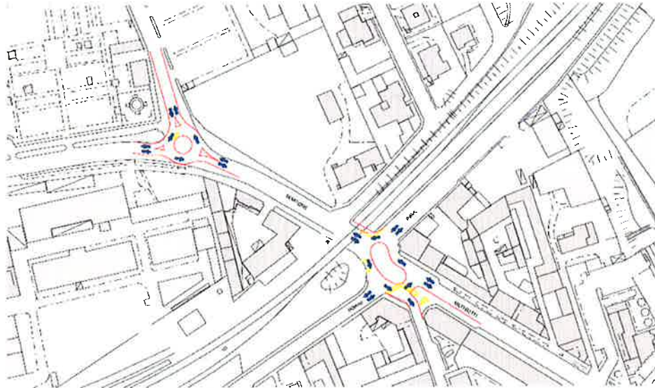
versione (1) elementi new jersey "mobili"
