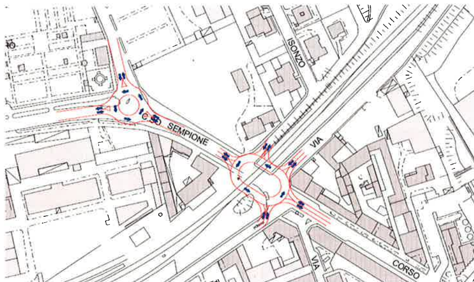
versione (2) elementi new jersey "fissi"
