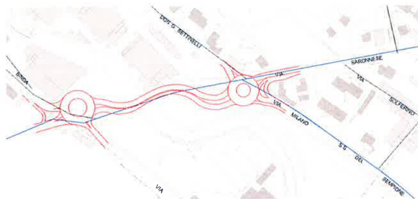
Sistema di rotonde SS. 527 ed SS. 33 (progetto realizzato)
